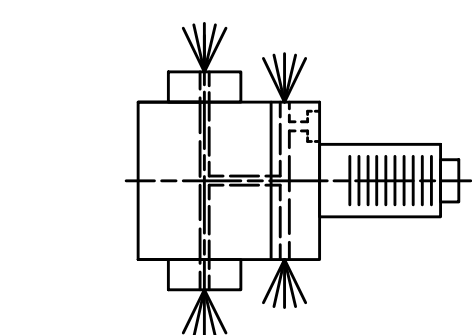
Innen- und Aussenkuehlung / Inside and outside coolant supply Kuehlmittelfiltrierung=50µ / coolant filtration=50µ
