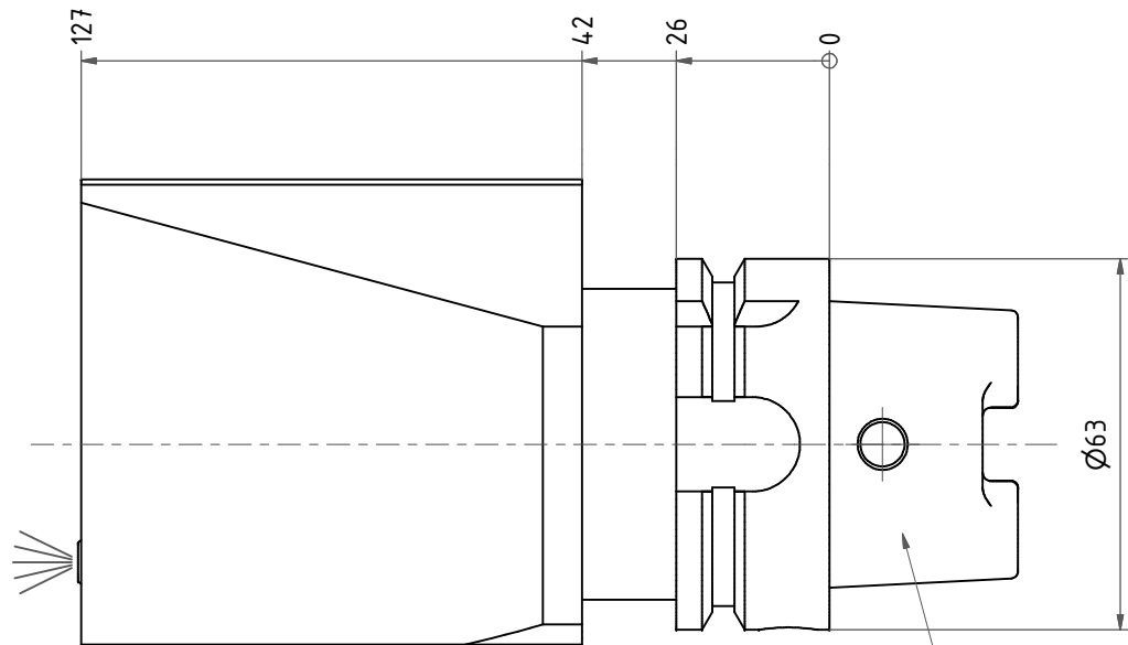
HSK 63A DIN 69893 Ausführung T
