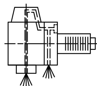
Innen- und Aussenkühlung / Inside and outside coolant supply Kuehlmittelfiltrierung-50µ / coolant filtration-50µ
