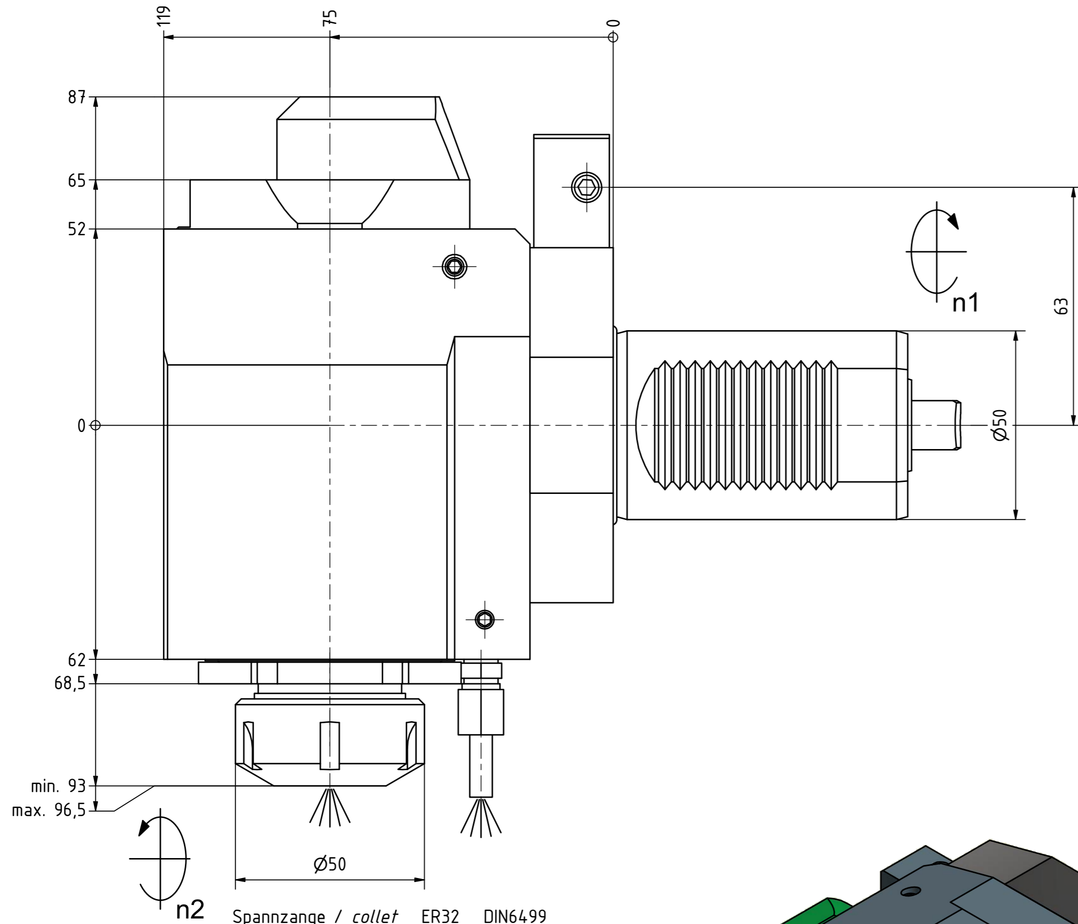
Spannzange / collet ER32 DIN6499 Spannbereich / clamping range: 2,0 - 20,0
