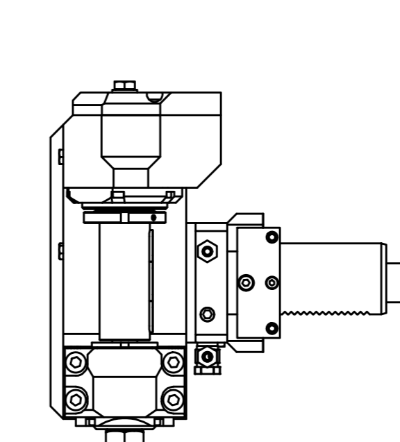
Doppelverzahnung Lizenz Traub double tooth system licence Traub
