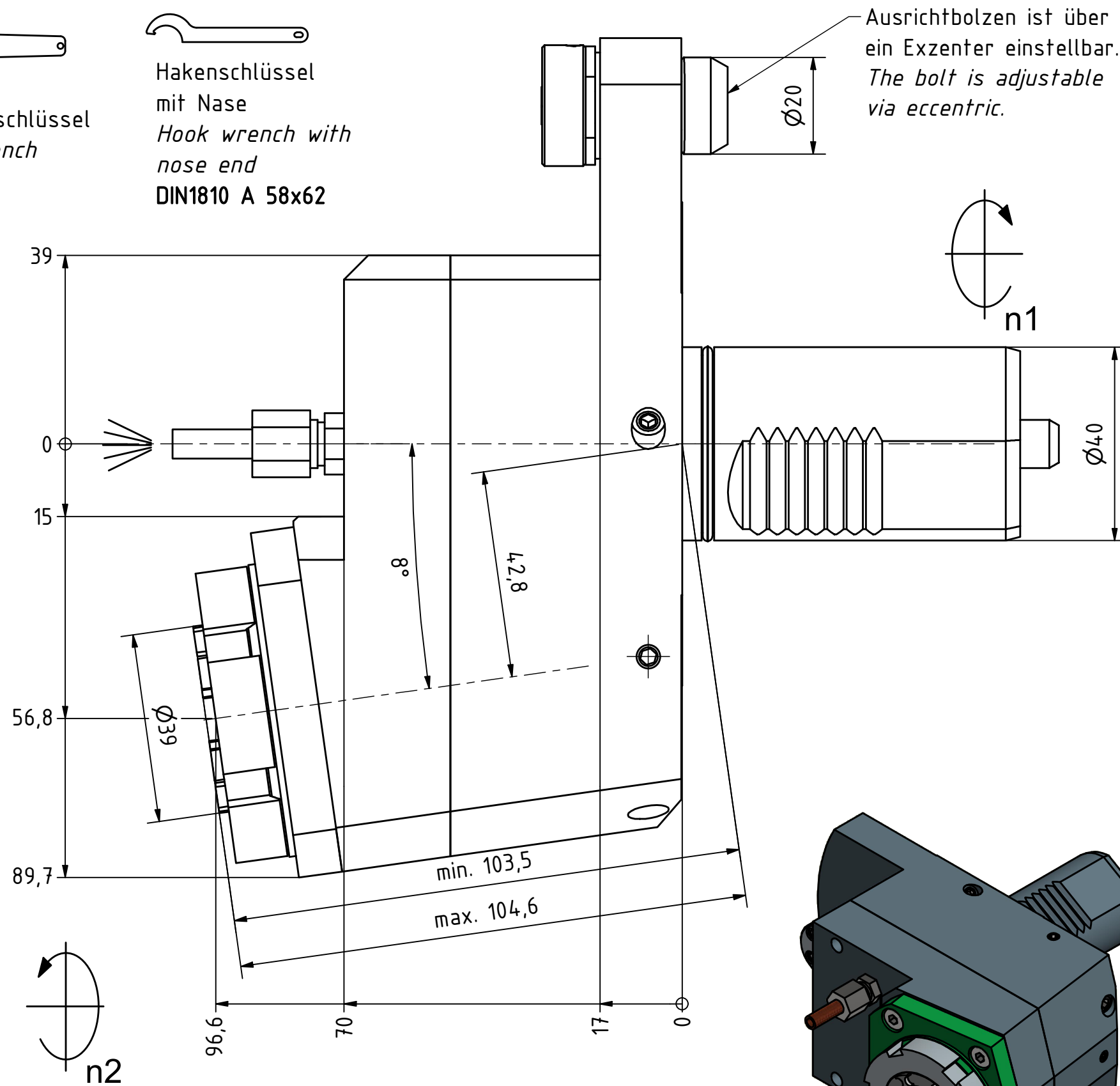
Spannzange / collet ER32 DIN6499 Spannbereich / clamping range: 2,0 - 20,0
