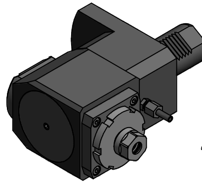
Spannzange / Collet ER16 DIN6499 Spannbereich / Clamping range: 1,0 - 10,0
