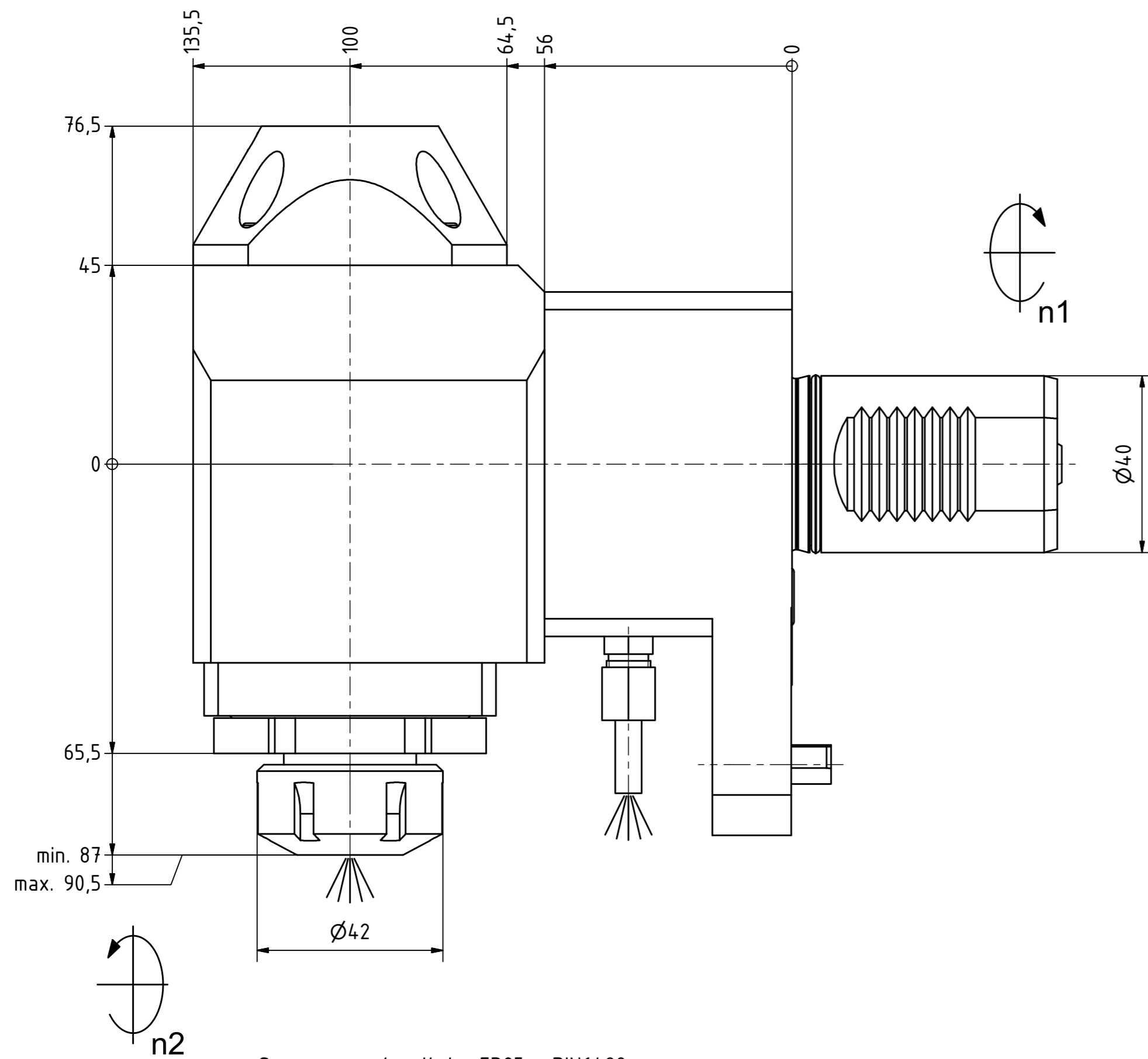
Spannzange / collet ER25 DIN6499 Spannbereich / clamping range: 1,0 - 16,0
