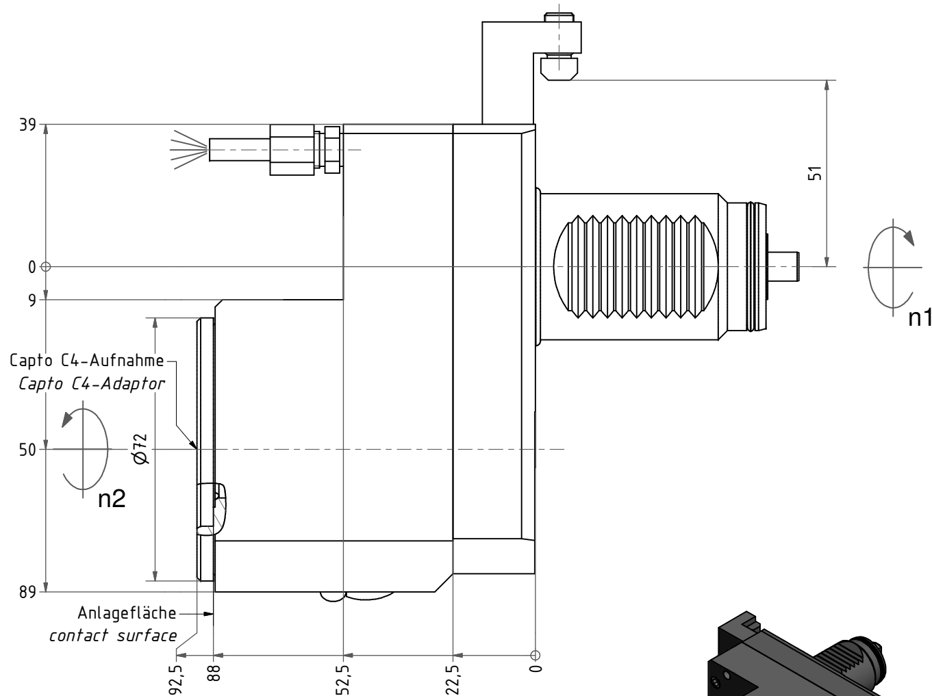
Capto C4-Aufnahme Capto C4-Adaptor
