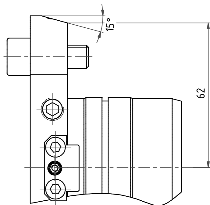
Ansicht X (1:1)
