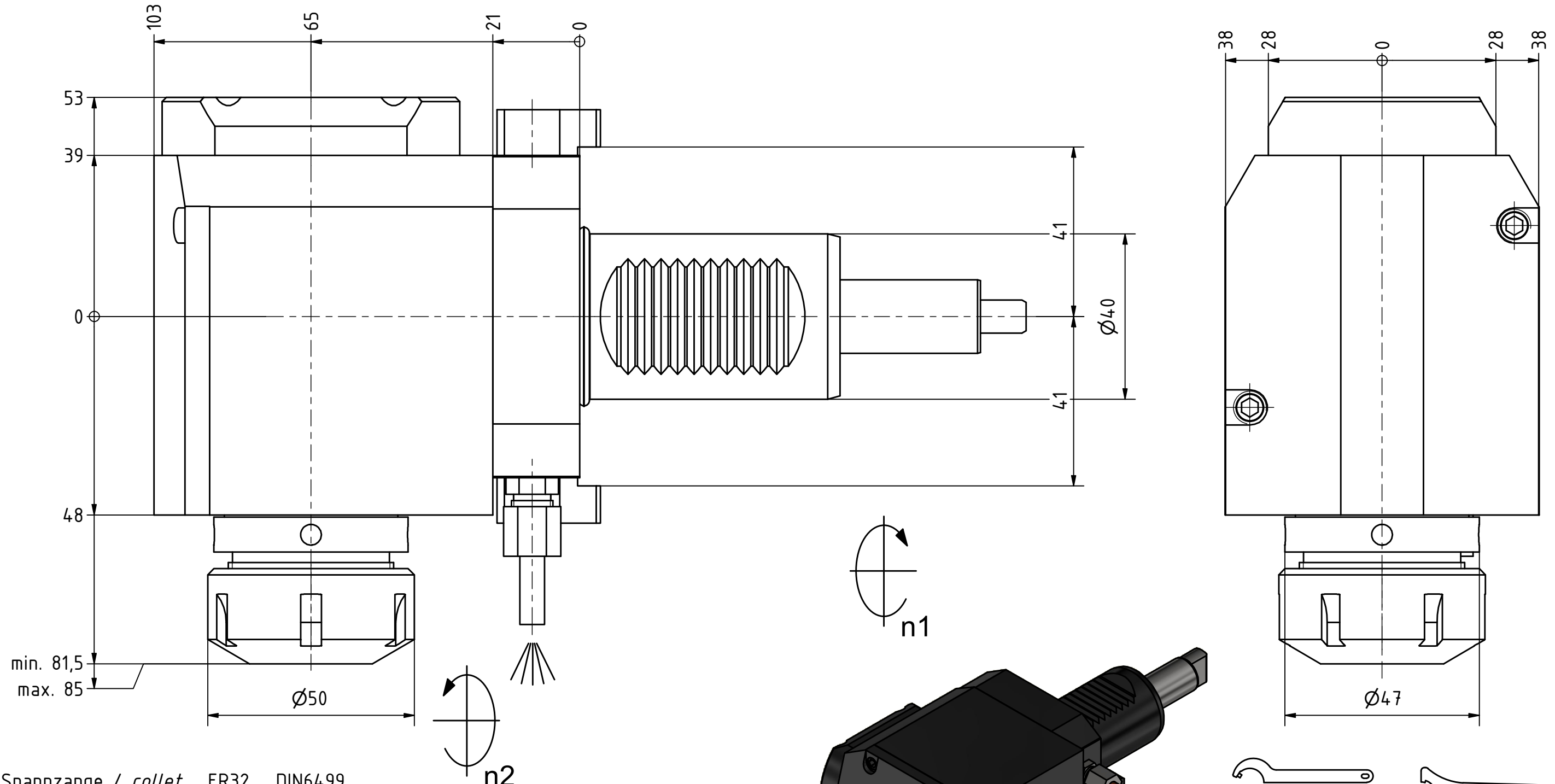
Hakenschlüssel mit Zapfen Hook wrench with fixed pin DIN1810 B 45x50 Spannzangenschlüssel Clamping wrench 232
