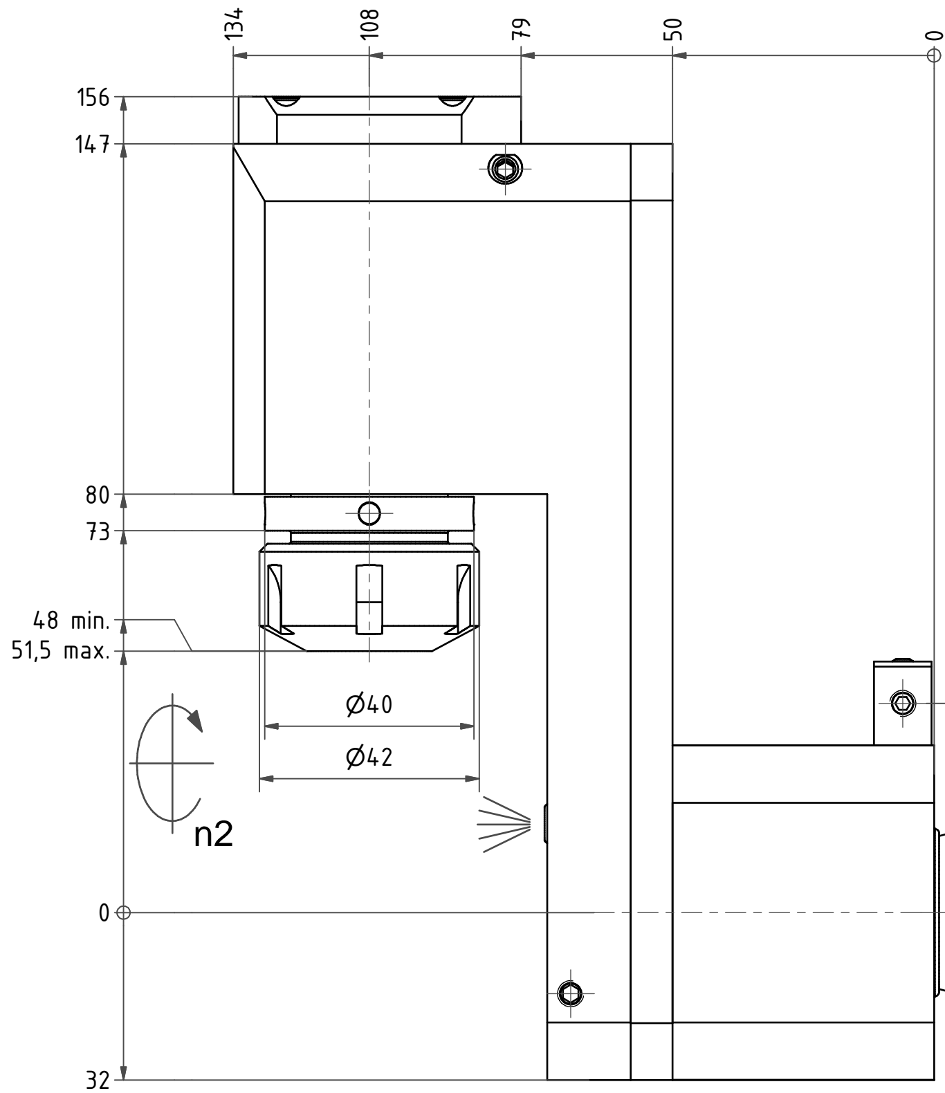
Spannzange / collet ER25 DIN6499 Spannbereich / clamping range: 1,0 - 16,0
