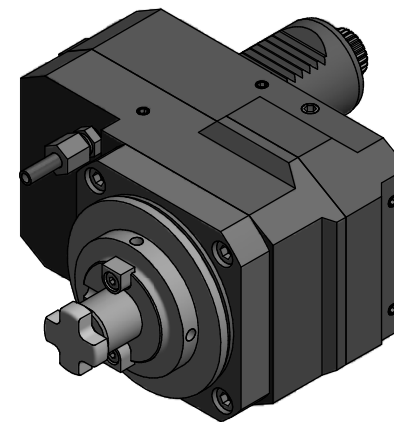
Bemerkung - Title Axial Fräskopf , achsversetzt Axial milling head offset
