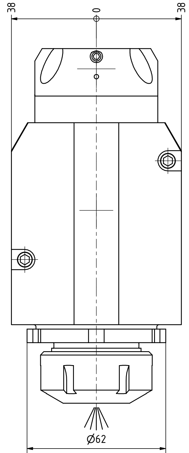
Spannzange / collet ER32 DIN6499 Spannbereich / clamping range: 2,0 - 20,0
