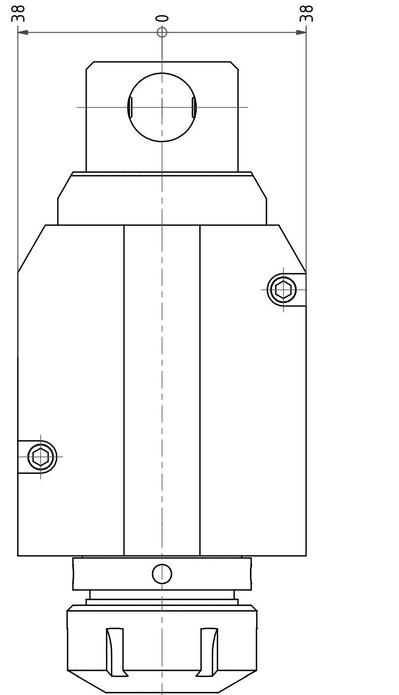
Hakenschlüssel mit Zapfen Hook wrench with fixed pin DIN1810 B 45x50 Spannzangenschlüssel Clamping wrench 232
