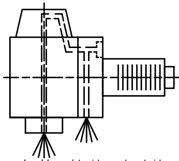
Innen- und Aussenkuehlung / Inside and outside coolant supply Kein Trockenlauf / No dry run Kuehlmittelfiltrierung <math>< 50\mu</math> / coolant filtration <math>< 50\mu</math>
