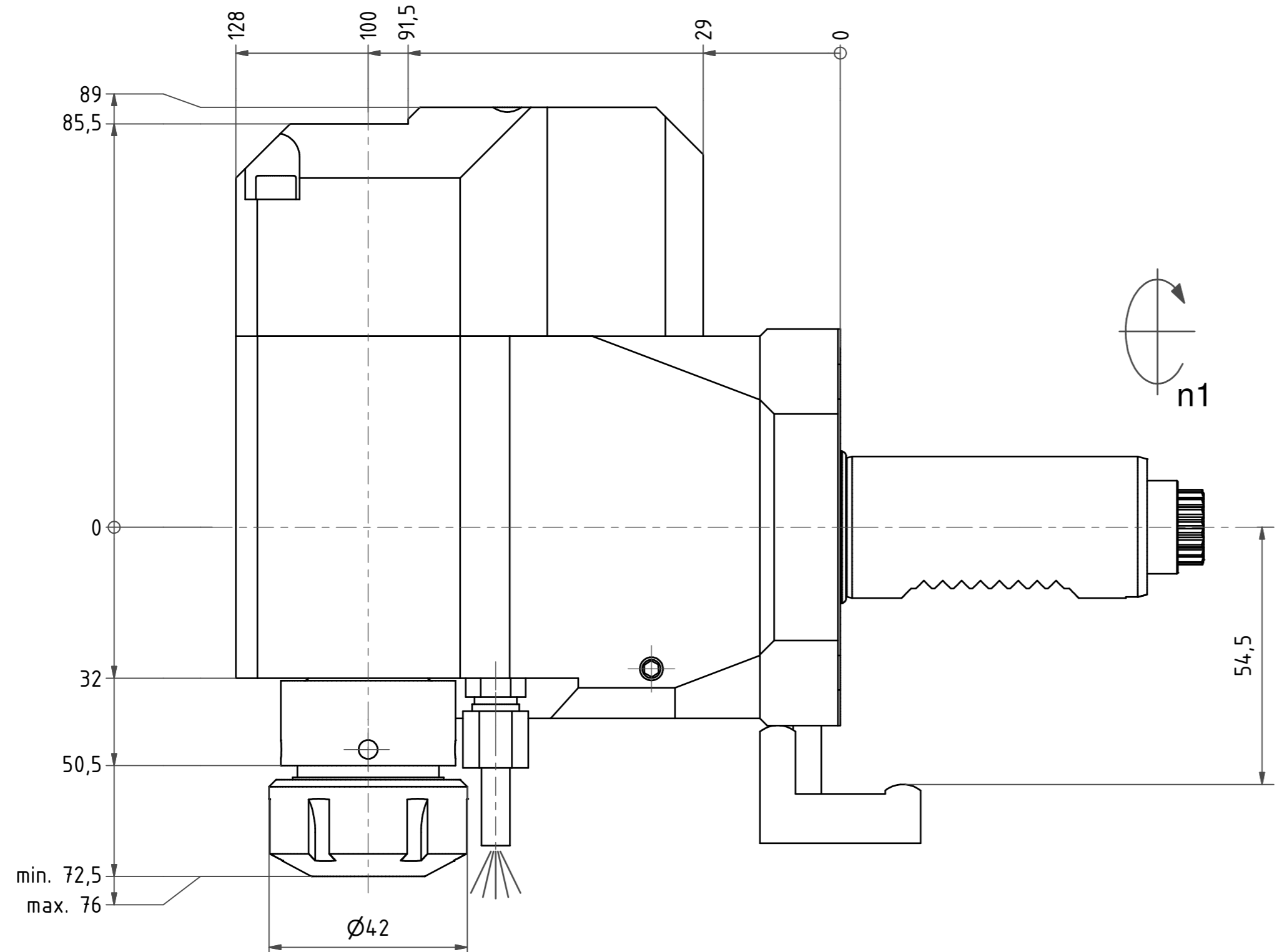
Spannzange / collet ER25 DIN6499 Spannbereich / clamping range: 1,0 - 16,0
