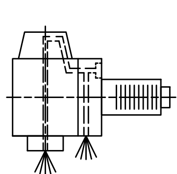
Innen- und Aussenkuehlung / Inside and outside coolant supply Kuehlmittelfiltrierung <math>50\mu</math> / coolant filtration <math>50\mu</math>
