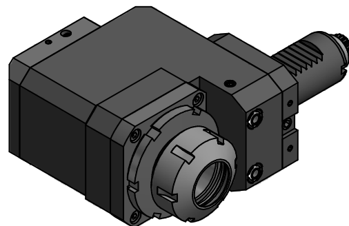
Spannzange / collet ER32 DIN6499 Spannbereich / clamping range: 2,0 - 20,0
