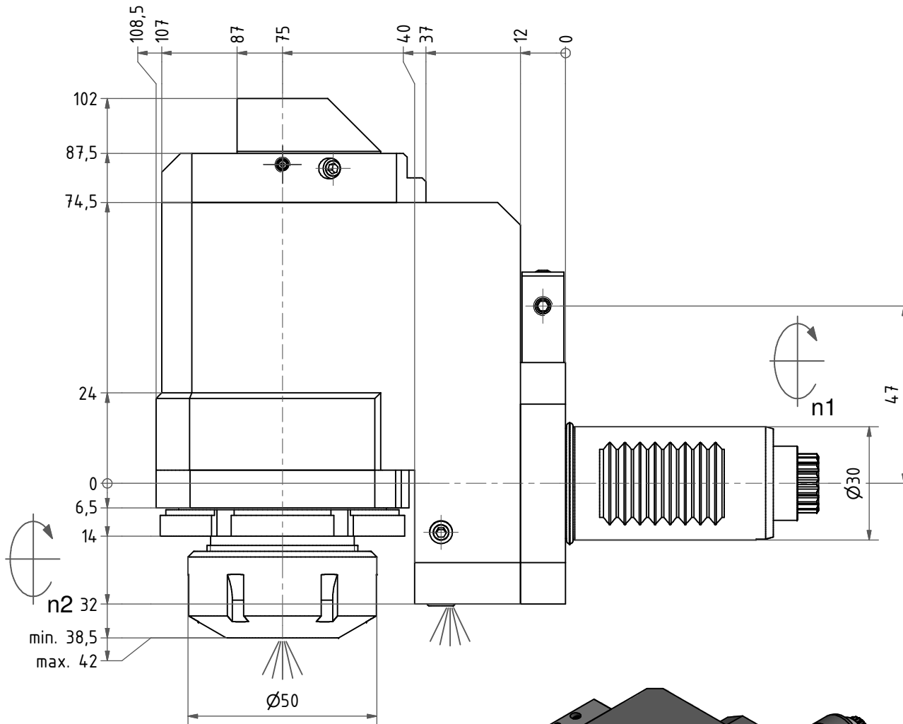
Spannzange / collet ER32 DIN6499 Spannbereich / clamping range: 2,0 - 20,0
