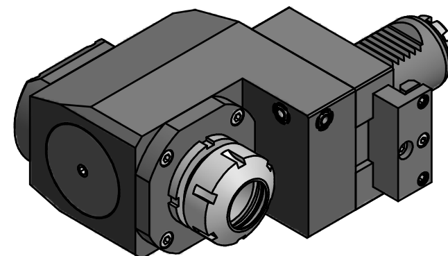
Doppelverzahnung Lizenz Traub double tooth system licence Traub
