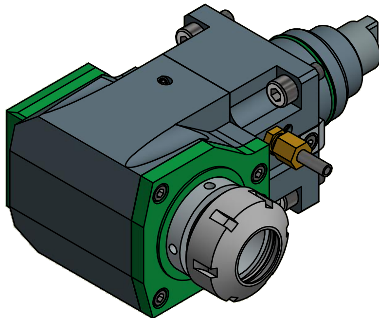
Spannzange / collet ER32 DIN6499 Spannbereich / clamping range: 2,0 - 20,0
