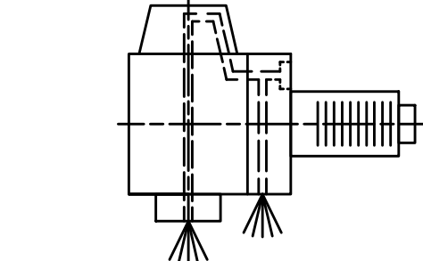
Spannzange / collet ER32 DIN6499 Spannbereich / clamping range: 2,0 - 20,0
