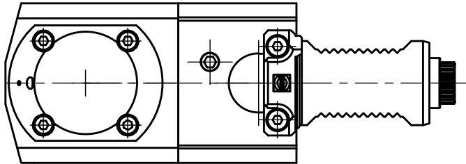
Doppelverzahnung Lizenz Traub double tooth system licenc Traub
