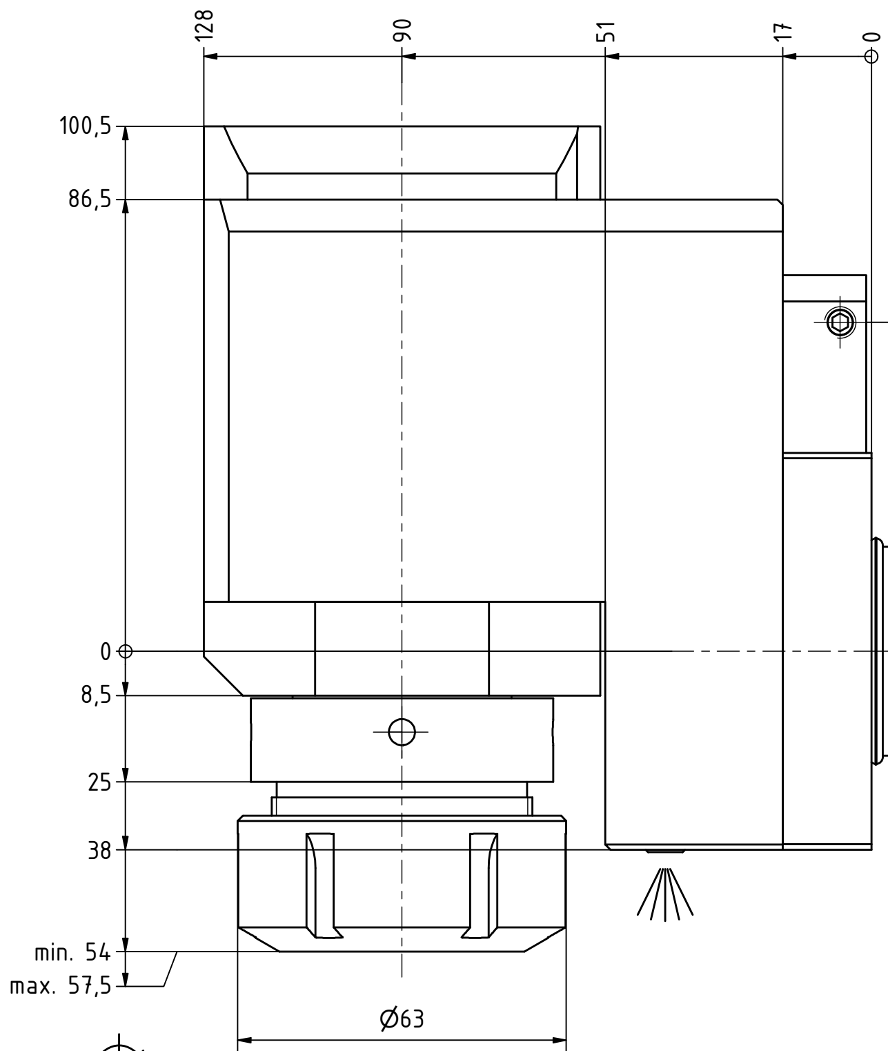
Spannzange / collet ER40 DIN6499 Spannbereich / clamping range: 3,0 - 26,0
