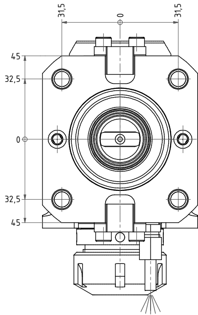
Spannzange / collet ER32 DIN6499 Spannbereich / clamping range: 2,0 - 20,0
