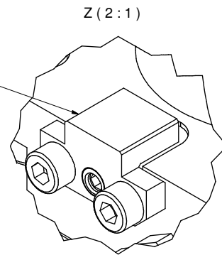
Ausrichtklotz ist über ein Exzenter einstellbar. The block is adjustable via eccentric.
