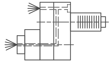
Innen- und Aussenkuehlung / Inside and outside coolant supply Kein Trockenlauf / No dry run Kuehlmittelfiltrierung <math>50\mu</math> / coolant filtration <math>50\mu</math>
