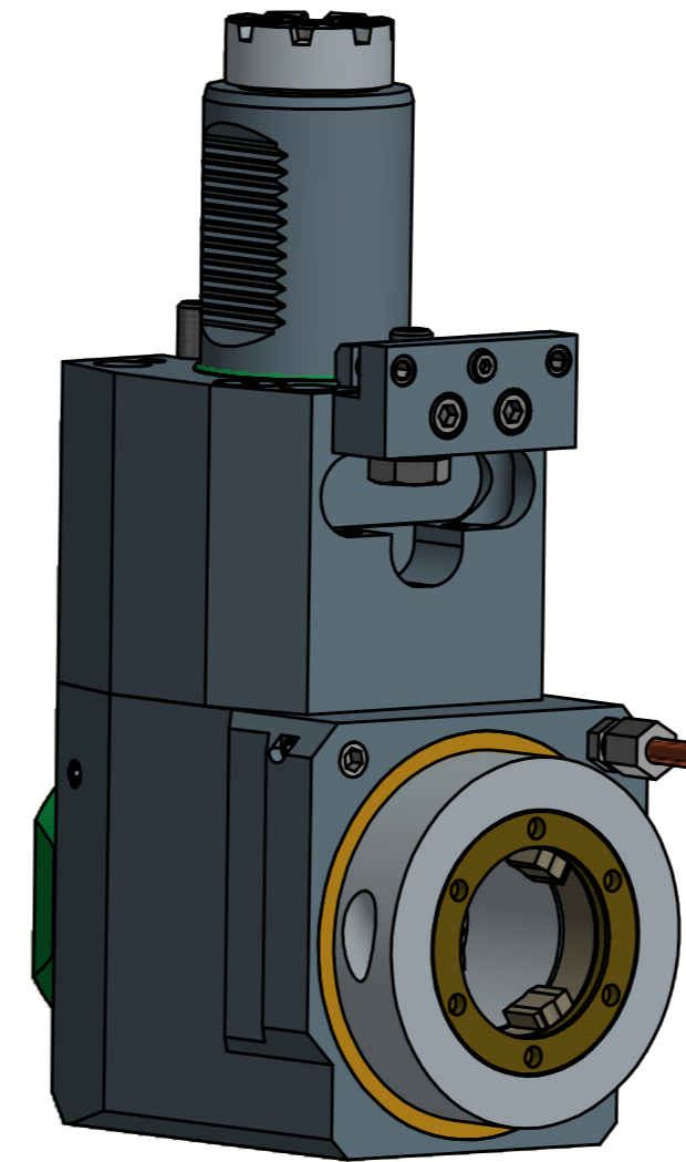
Innen- und Aussenkuehlung / Inside and outside coolant supply Kuehlmittelfiltrierung-50µ / coolant filtration-50µ
