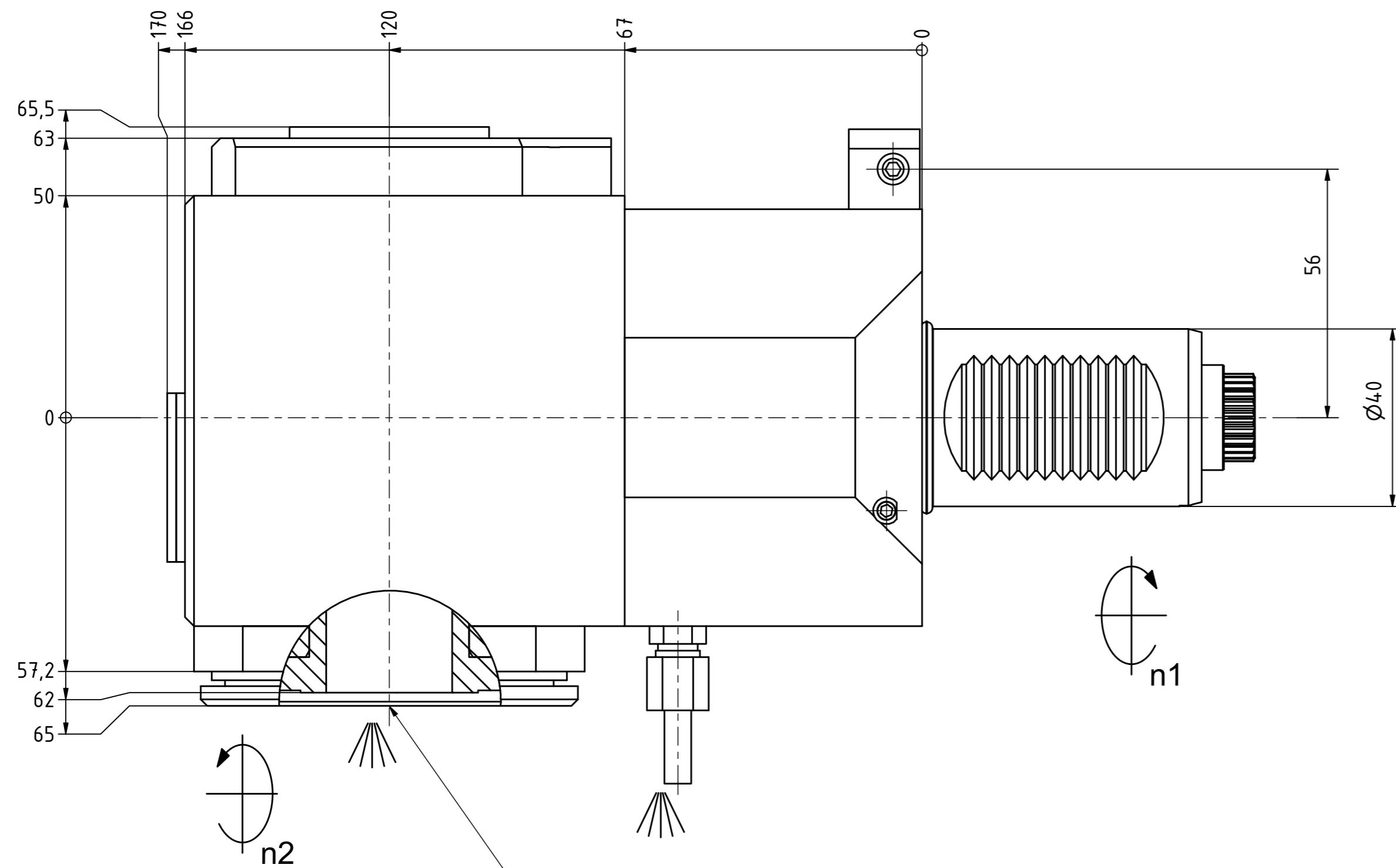
Capto C4-Aufnahme Capto C4-Adaptor
