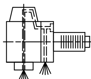
Innen- und Aussenkühlung / Inside and outside coolant supply Kuehlmittelfiltrierung=50µ / coolant filtration=50µ
