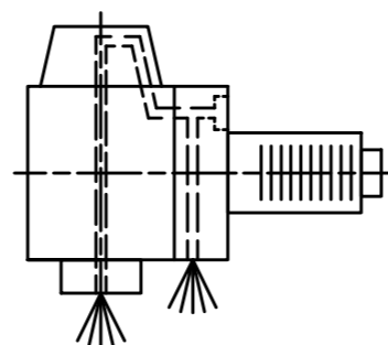
Innen- und Aussenkuehlung / Inside and outside coolant supply Kuehlmittefiltrierung=50µ / coolant filtration=50µ
