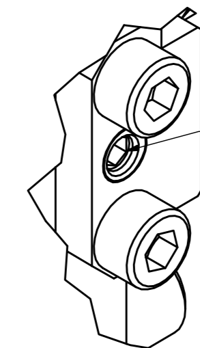
Ausrichtklotz ist über ein Exzenter einstellbar. The block is adjustable via eccentric.
