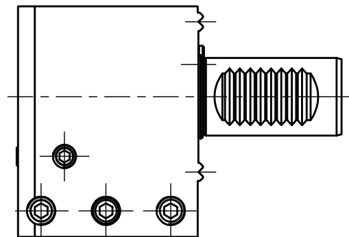
( 1 : 2 ) W-Verzahnung Lizenz Index-Werke W-tooth system licence Index-Corporation
