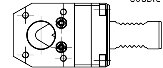
( 1 : 2 ) Doppelverzahnung Lizenz Traub double tooth system licence Traub
