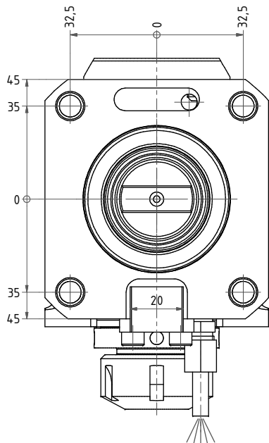
Spannzange / collet ER25 DIN6499 Spannbereich / clamping range: 1,0 - 16,0
