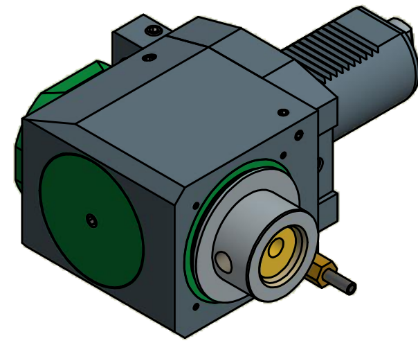
KM 40-Aufnahme KM 40-Adaptor
