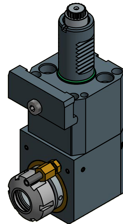
Doppelverzahnung Lizenz Traub double tooth system licence Traub
