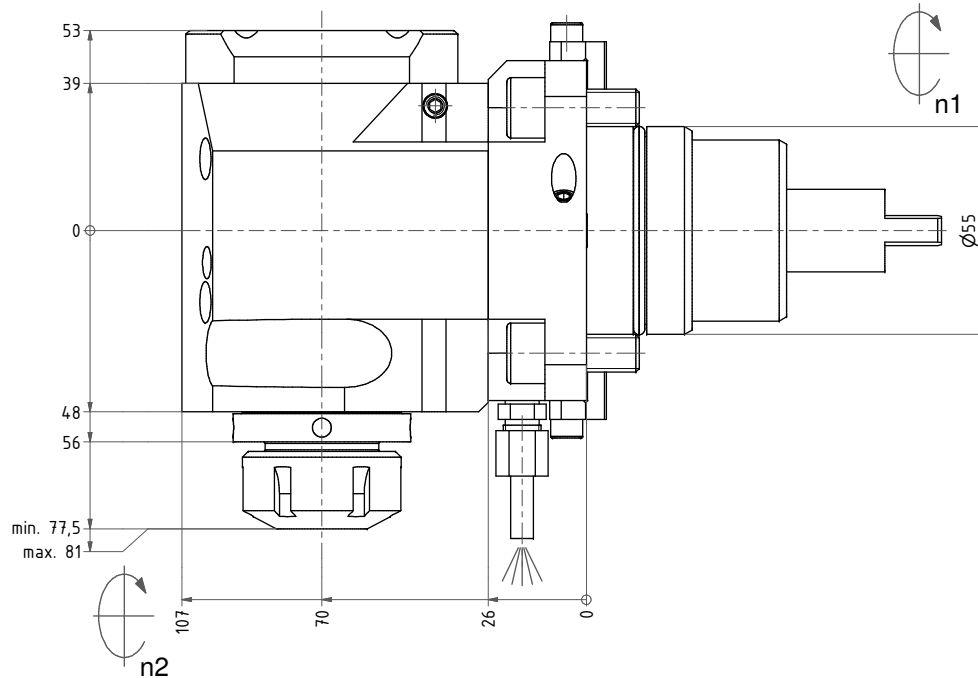
Z (2 : 1)
