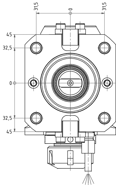
Spannzange / collet ER25 DIN6499 Spannbereich / clamping range: 1,0 - 16,0
