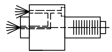
Innen- und Aussenkuehlung / Inside and outside coolant supply Kuehlmittelfiltrierung <math>< 50\mu</math> / coolant filtration <math>< 50\mu</math>
