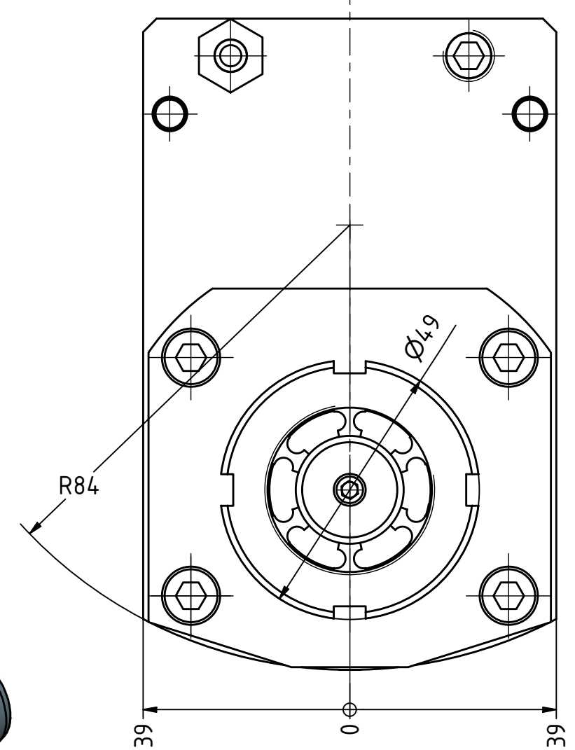
Spannzange / collet ER25 DIN6499 Spannbereich / clamping range: 1,0 - 16,0
