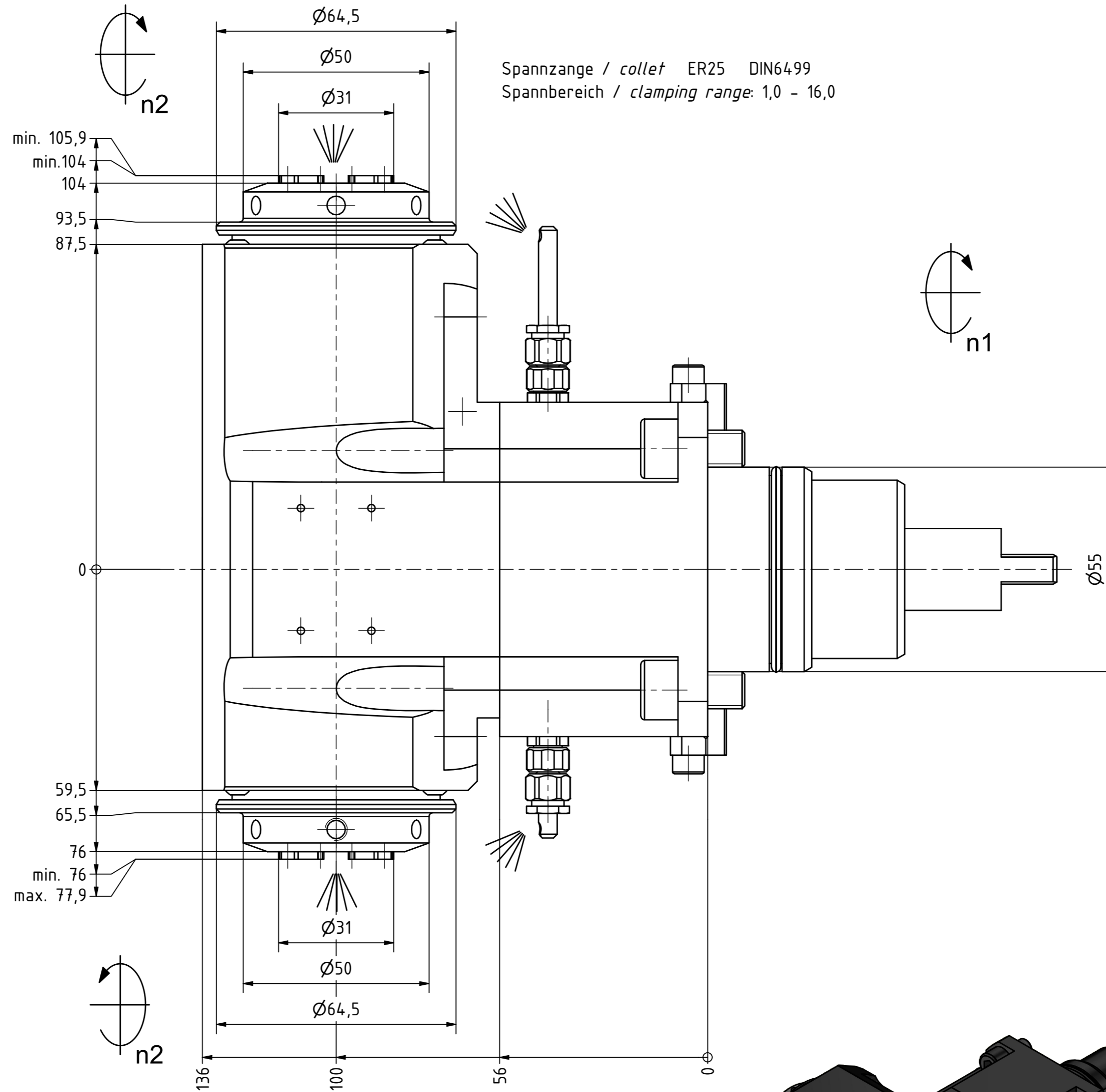
Spannzange / collet ER25 DIN6499 Spannbereich / clamping range: 1,0 - 16,0
