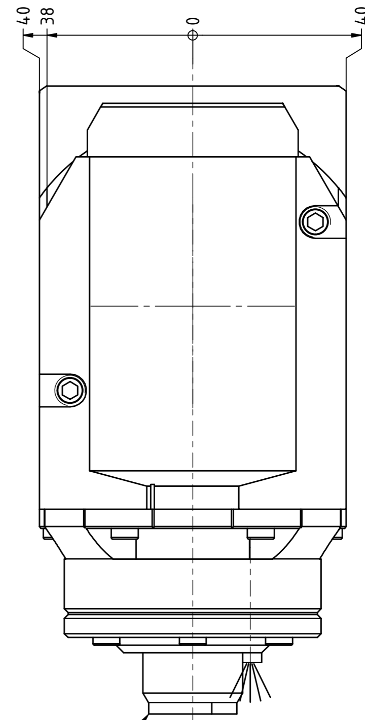
Formbore-Kopf MF1 Formbore-Head MF1
