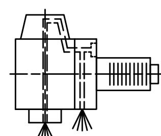
Innen- und Aussenkühlung / Inside and outside coolant supply Kühlmittelfiltration=50µ / coolant filtration=50µ
