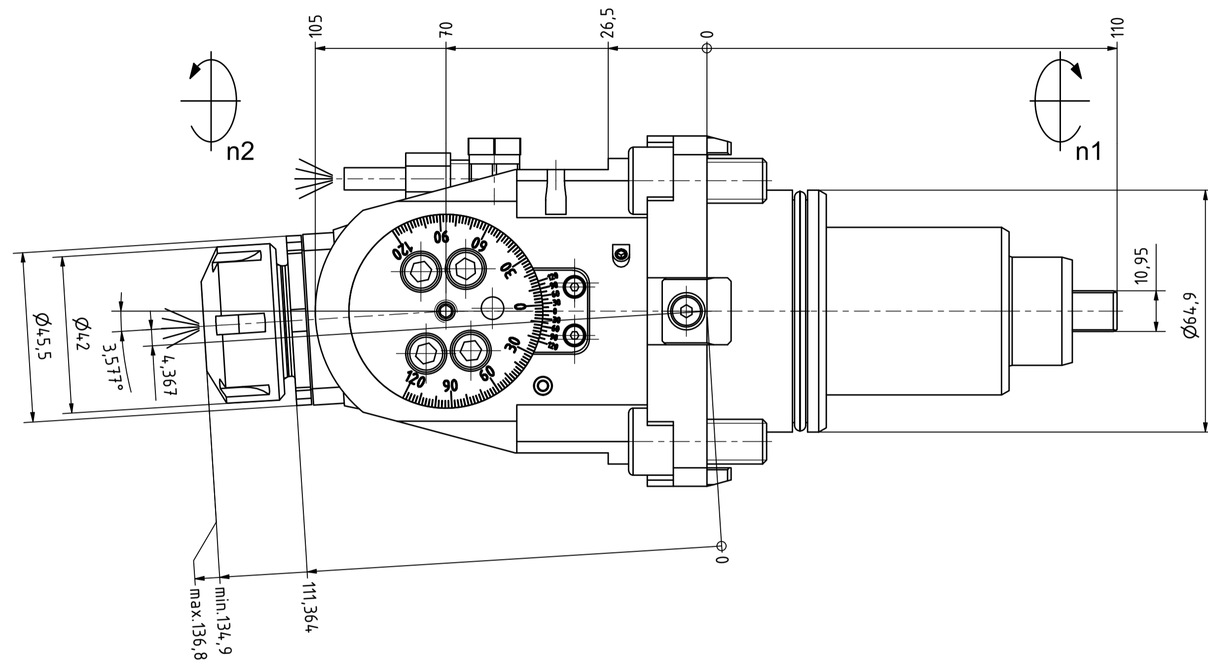
Spannzange / collet ER25 DIN6499 Spannbereich / clamping range: 1,0 - 16,0
